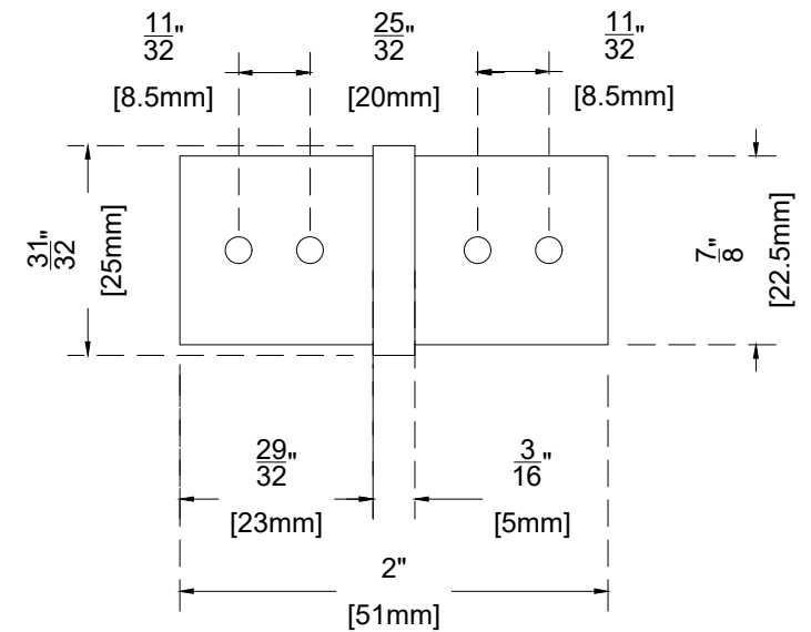
VUE EN PLAN - plan view
