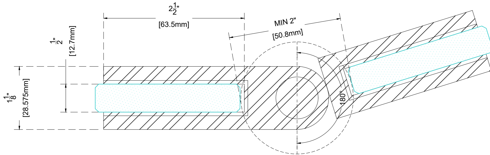
VUE EN PLAN - plan view
