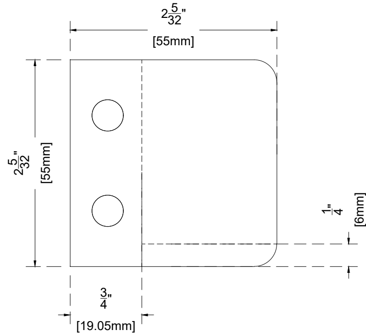
VUE DE FACE- AVEC PLAQUE front view with bottom plate
