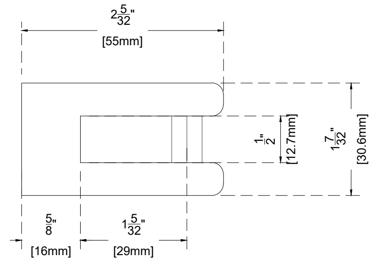
VUE EN PLAN- plan view
