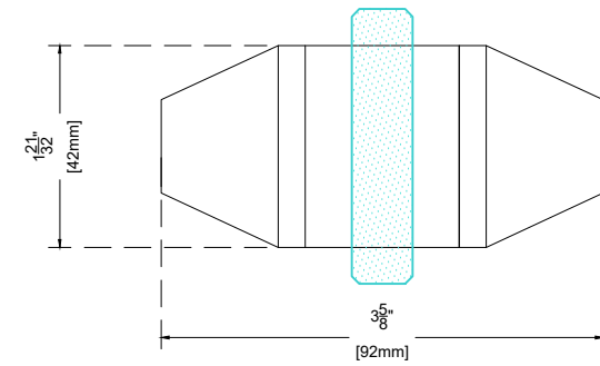
VUE EN PLAN - plan view
